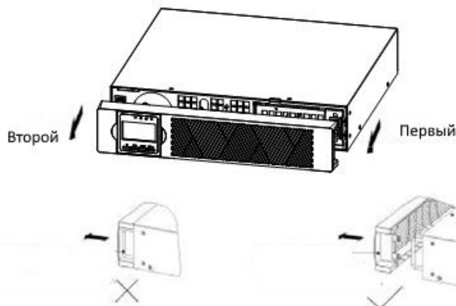
Рисунок 8 – Снятие передней крышки батарейного модуля
