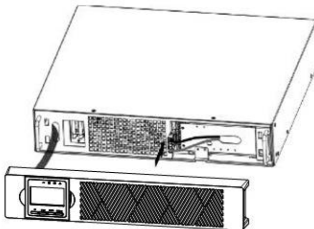
Рисунок 6 – Подключение внутренних батарей
