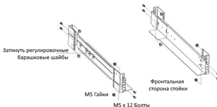
Рисунок 2 – Крепление монтажного комплекта рельс
