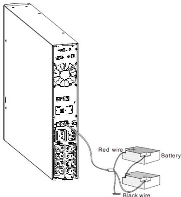
Рисунок 11 – Подключение внешних аккумуляторов
