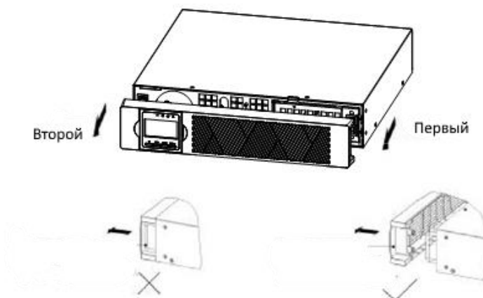
Рисунок 5 – Снятие передней крышки ИБП
