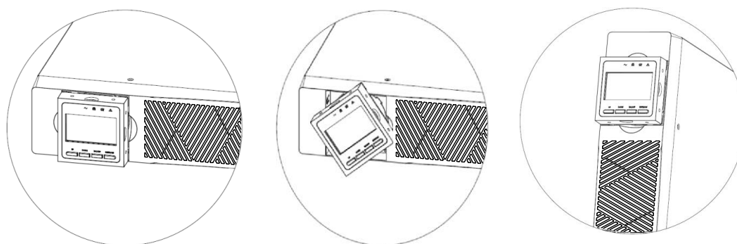
Рисунок 14 – Установка дисплея для вертикального использования
