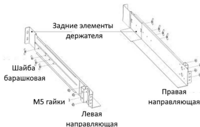
Рисунок 1 – Крепление монтажного комплекта рельс
