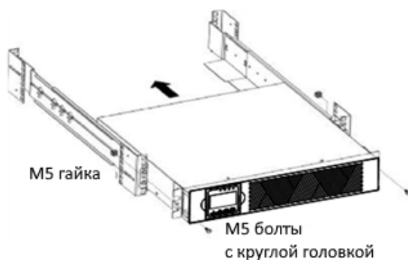
Рисунок 4 – Установка и крепление ИБП в стойке
