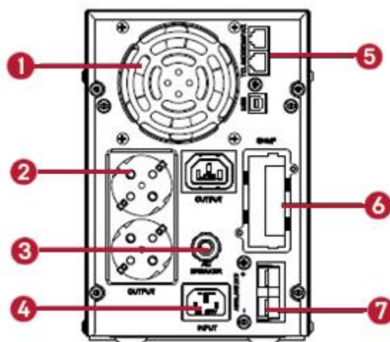
Вид задней панели ИБП
